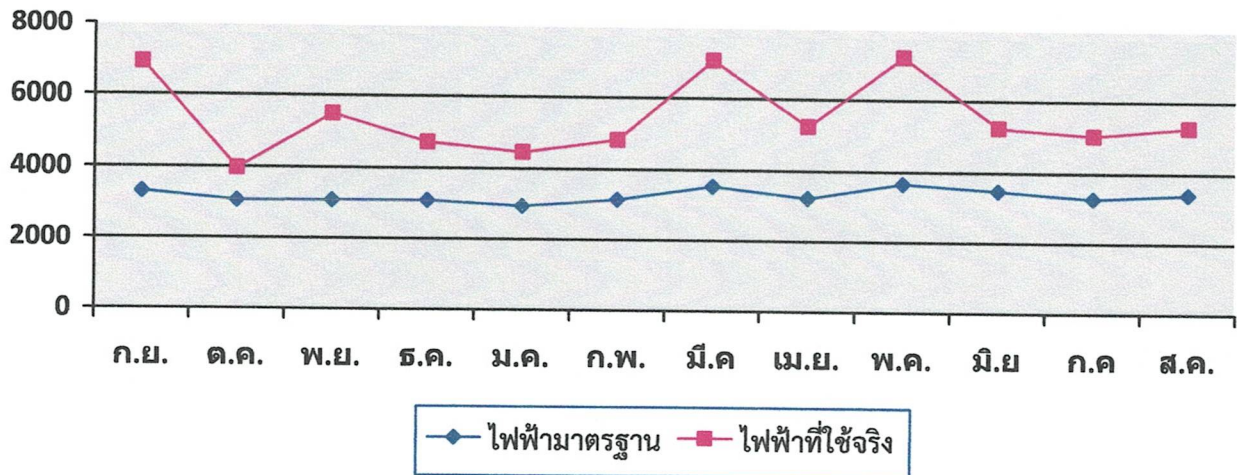
ตารางเปรียบเทียบค่ามาตรฐานการใช้พลังงานไฟฟ้า(หน่วย) และการใช้พลังงานจริง
